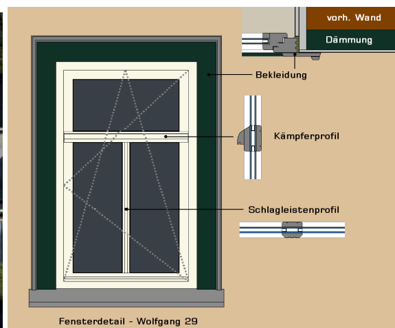
Fensterdetail
